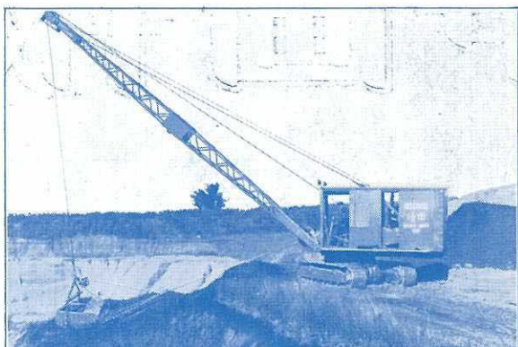
米國ウイソコンシン洲デエームスビール市、シキユーリテ、ウアシユド、サンド、エンド、グラベル會社の砂利坑にて働きつゝある堅牢なる、オスグード11碼瓦斯倫ドラグライン。
