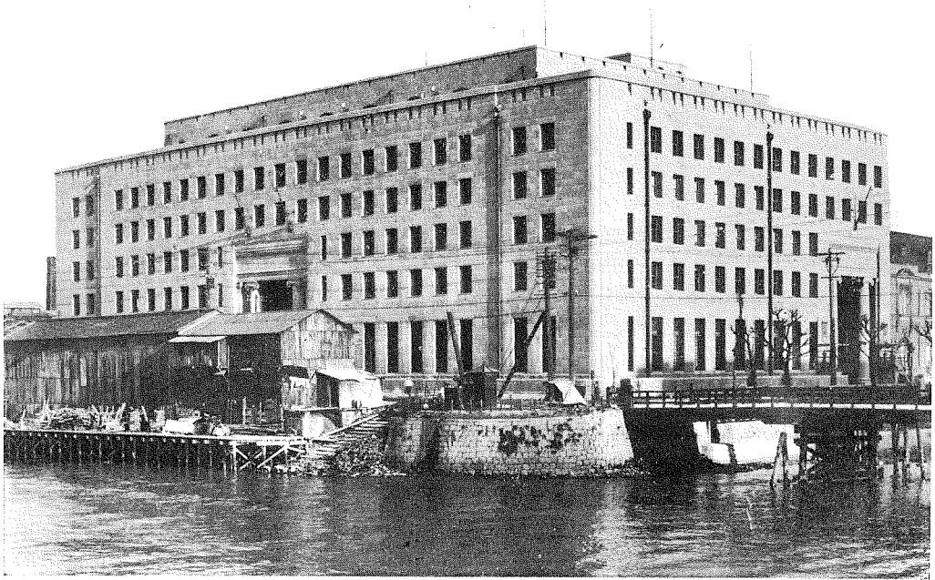
最近竣工したる大阪住友ビルディングの大建築 New Sumitomo Building, Recently Completed. Osaka, Japan.
