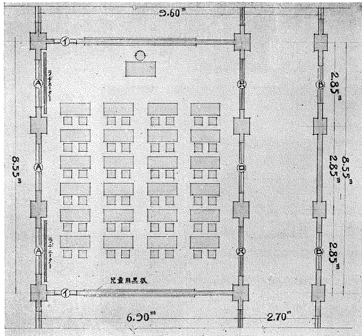
(8) 東京市立小學校平面規格圖 (8) Plan of Class Room and Hall Way.
