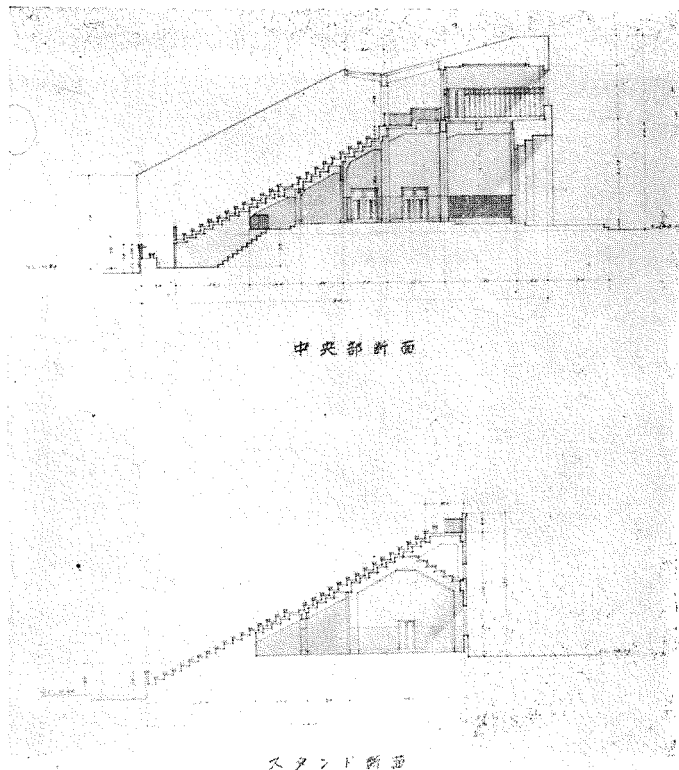
(6) 断面 圖
