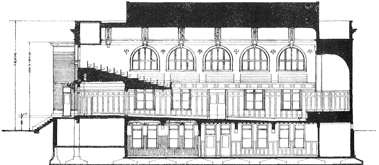
縦 断 面 圖
