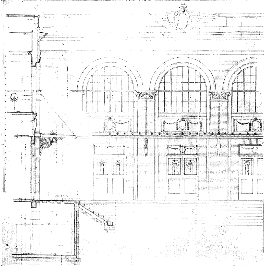
(3) 正面詳細圖
