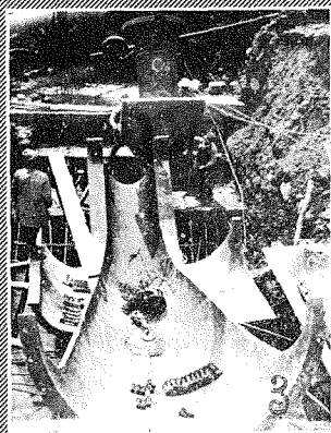
(7) パースチングピット施工圖 (1)假組立、(2)掘鑿及基礎工、(3)据付中 (4)据付中、(5)据付中、(6)据付終リコン クリートにて被覆す。(信越電力)
