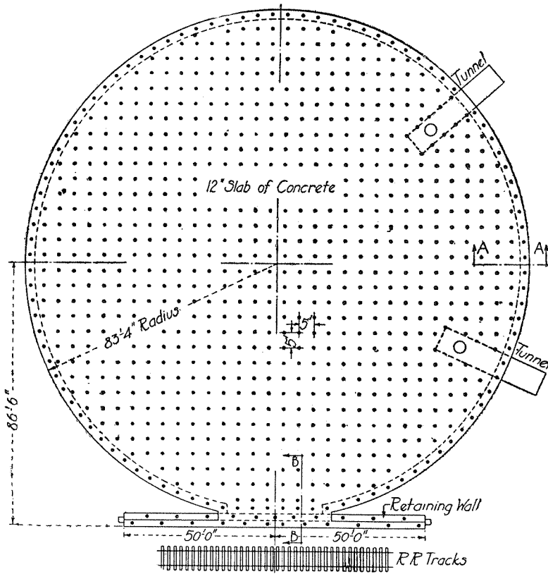
タンクの基礎圖
