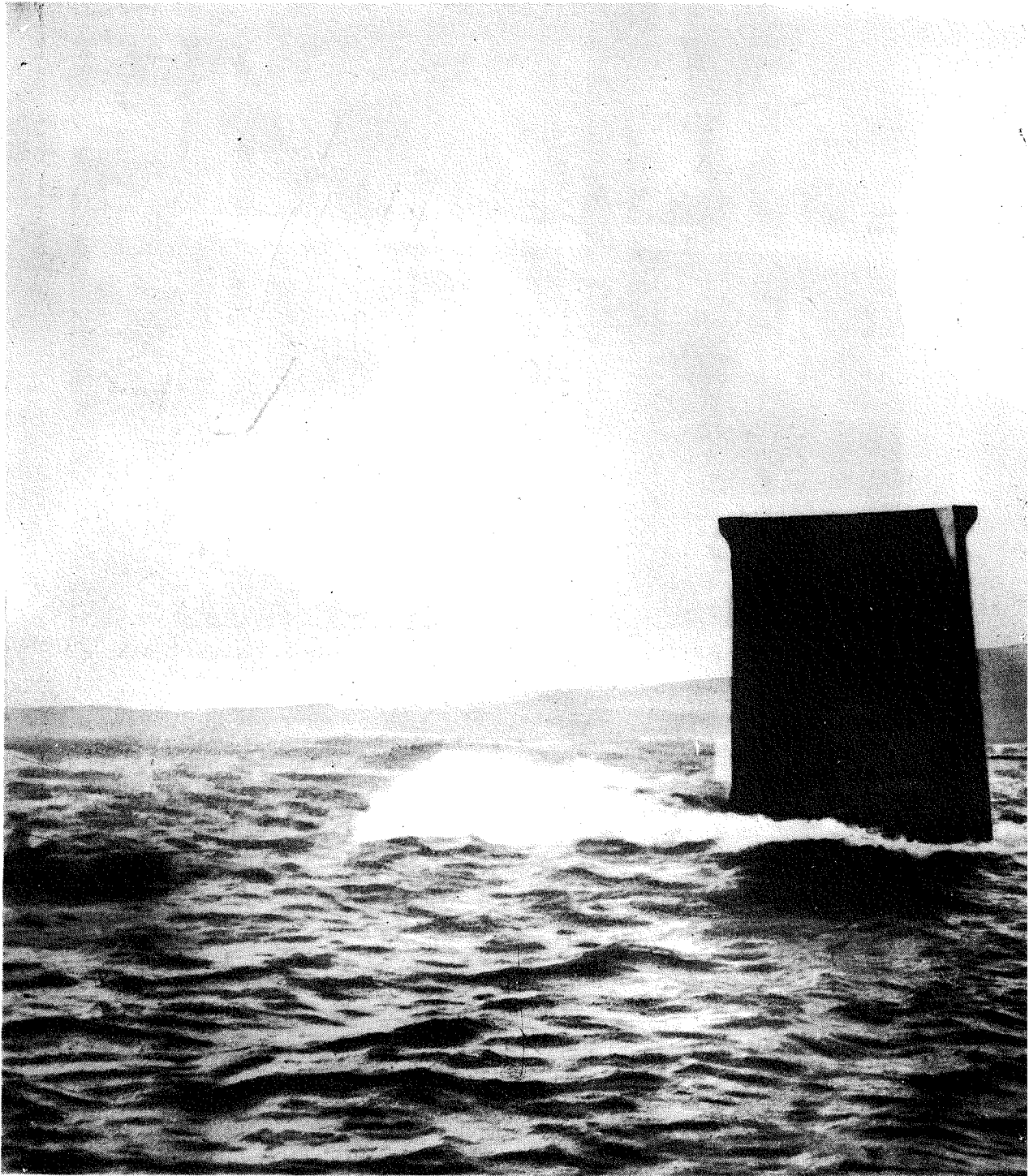
鐵道省青函聯絡設備改良工事（函館） 進水中の「ケーソン」 進水後は吃水量約21呎となり浮揚のまま据付箇所迄運搬す。 大正十三年七月
