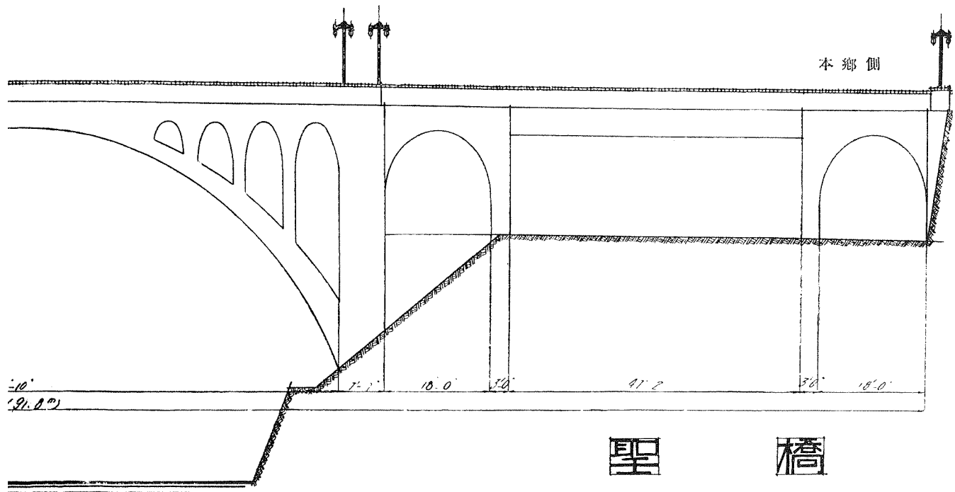
断面圖
