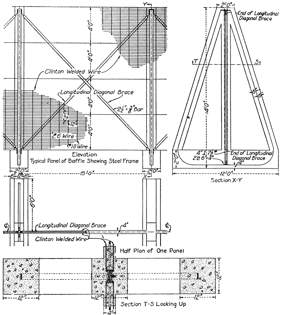
前圖ウォールの設計圖
