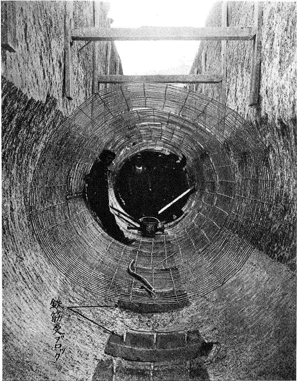
鐵筋敷設の段取
