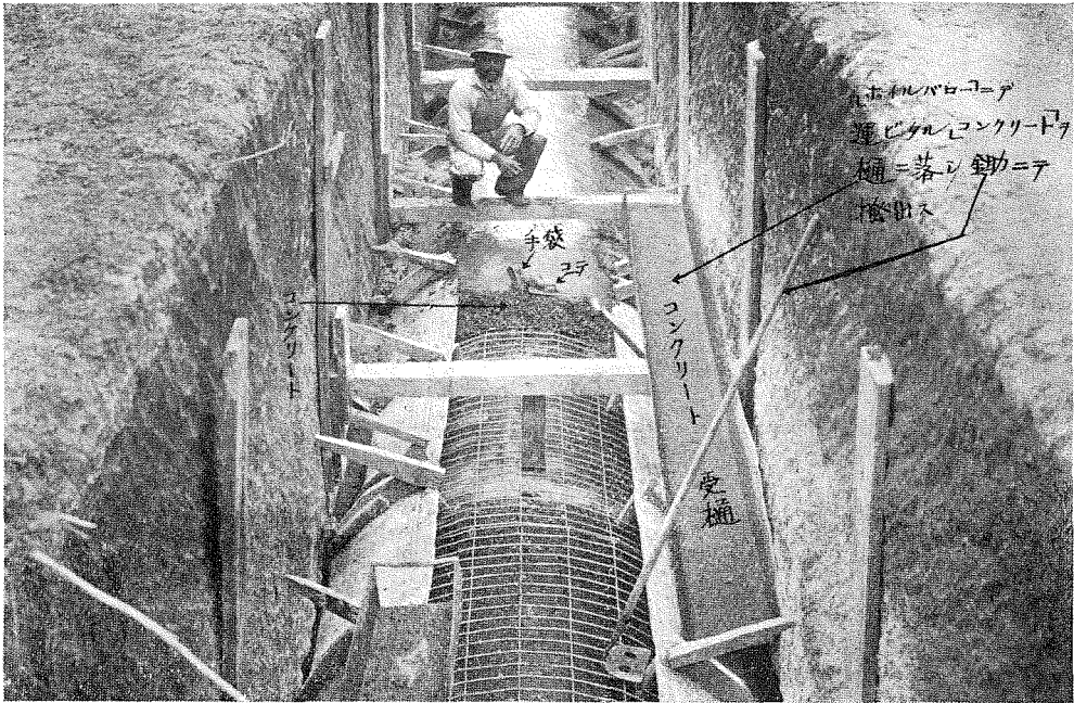
段取りき下水管工事
