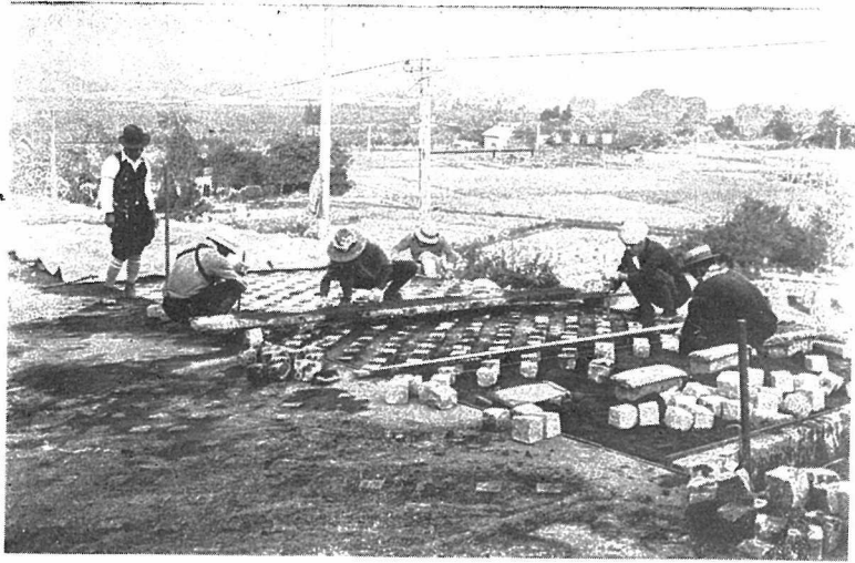
府縣道飯坂福島線 福島縣信夫郡飯坂町地内 工法二層式混凝土鋪裝工鋪裝幅員 6.0 米 平均厚 20 糎 下層 1:3:6 平均厚 15 糎 上層 1:1.5:3 厚 5 糎 急坂部小鋪石滑止鋪裝工小鋪石 9 糎立方一平方米當リ 24 個使用
