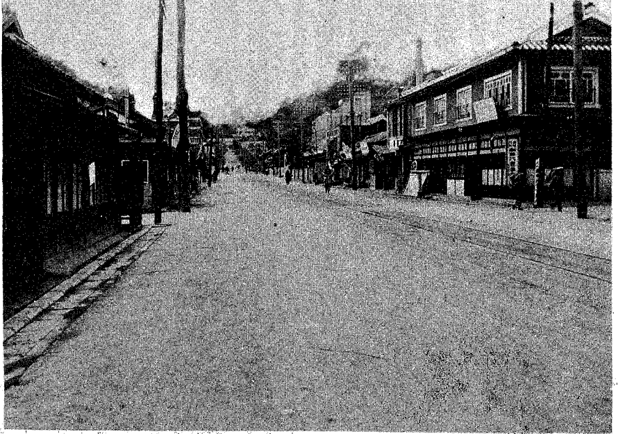
朝鮮釜山府大廳町アスファルト舗装道路(トベカ式五糎厚) 昭和八年十月竣工 日本石油株式會社道路部施工
