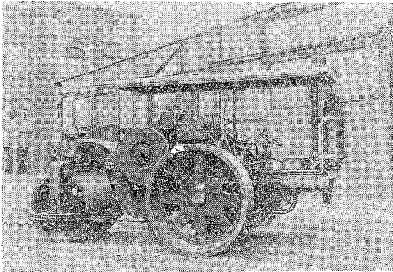
「ケムナ」拾噸マカダム型デイズルロードローラー
