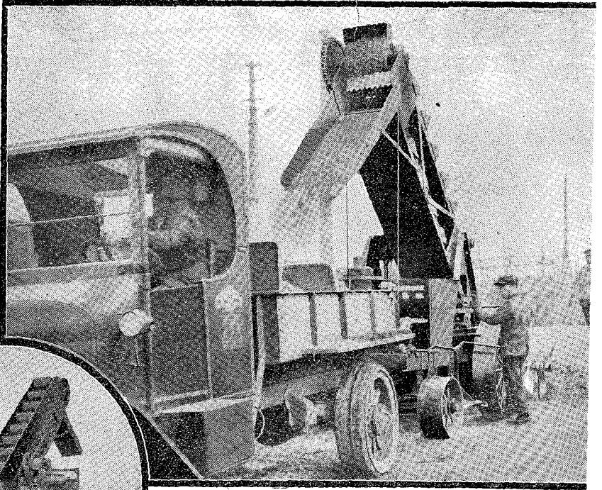
日本石油株式会社納入ヘース積込機
