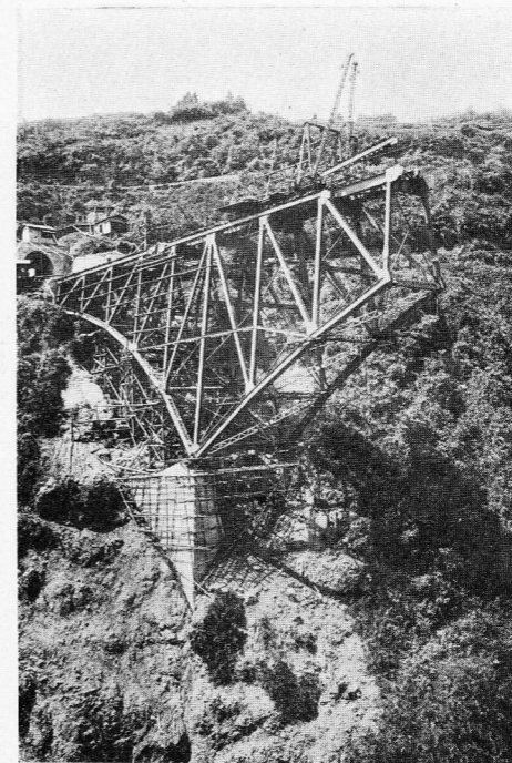
立野側中央径間アッパー・コード組立
