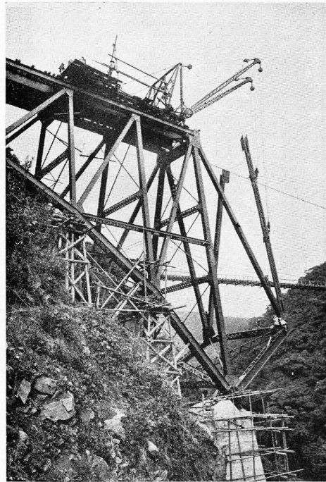
立野側中央径間ヴァーチカル建込み
