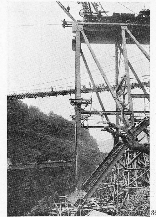
高森側中央径間ローワー・コード組立
