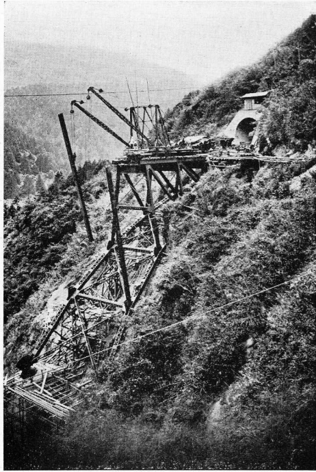
立野側径間ヴァーチカル建込み
