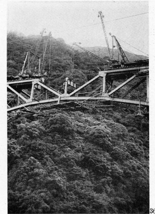
中央フローア・ビーム取付
