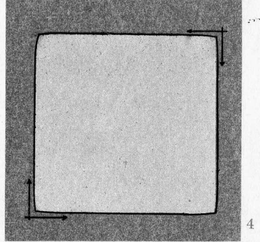
一様なる剪力を与へたる場合
