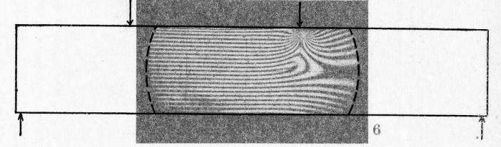
一様なる弯曲率を与へたる場合
