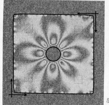
一様なる弯曲率を与へたる場合
