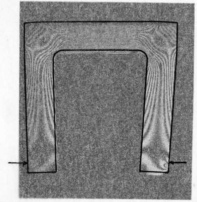
框構の場合
