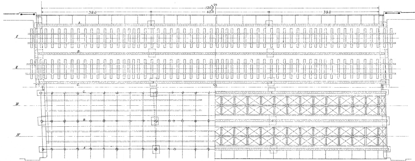
平面圖
