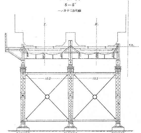
橫斷面
