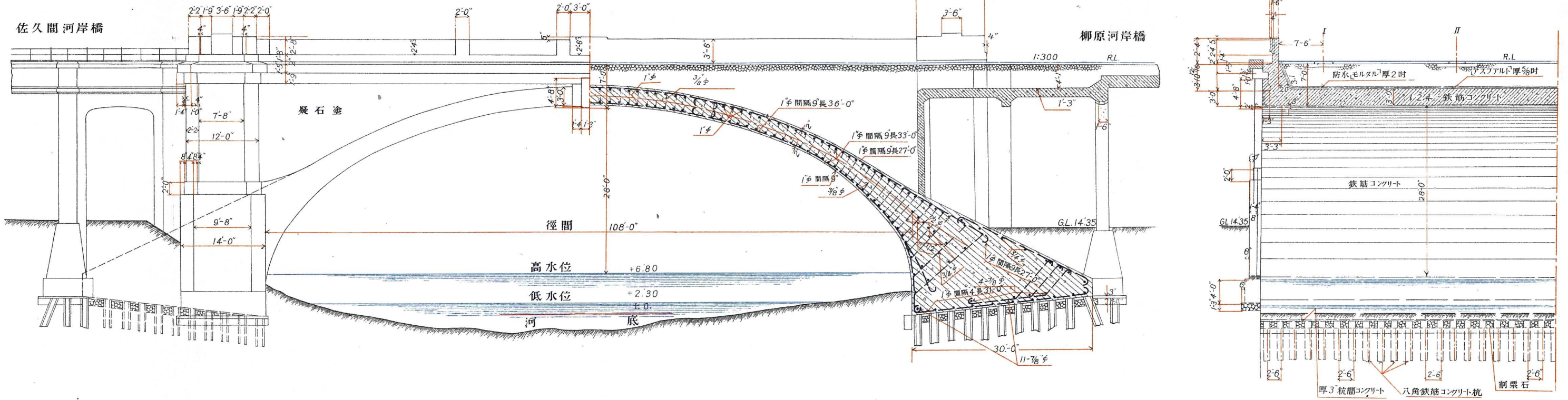
横斷面圖
