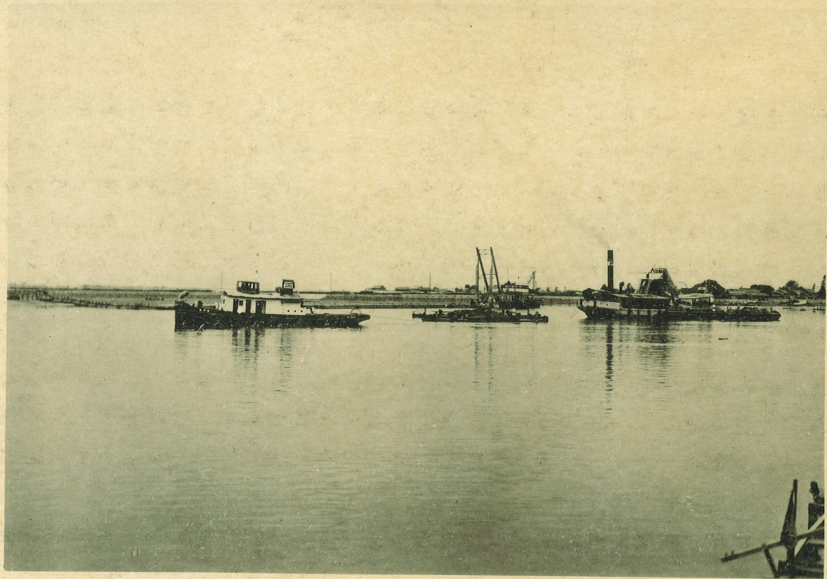
旭川（福島地先）浚渫作業 左 曳船旭川丸 ディーゼルエンジン 150馬力 8海里堀 中央 電動ポンプ式浚渫船 旭號 3000立米堀 右 助籠式浚渫船 安治川丸 1200立米堀
