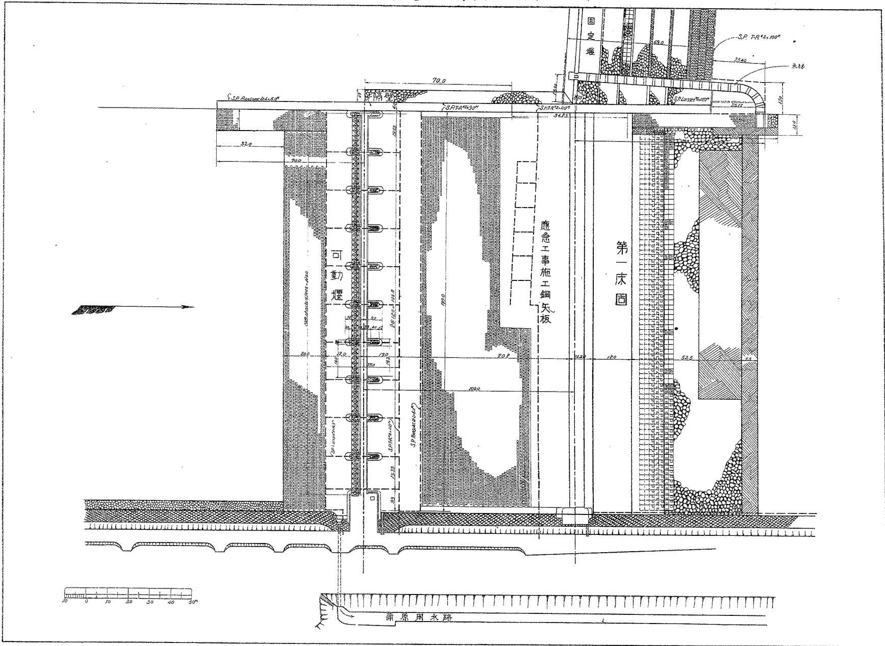
可動堰及第一床固平面圖
