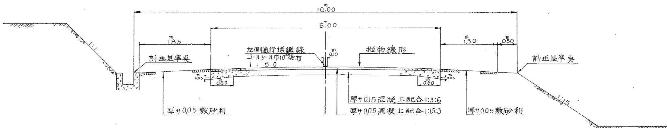
郊外地横断面定規圖
