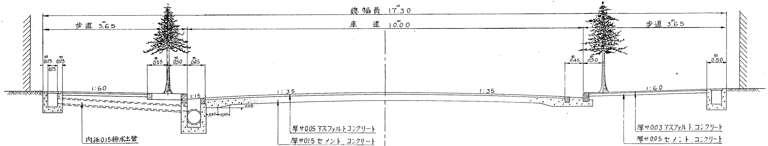
明后市内横断面定規圖
