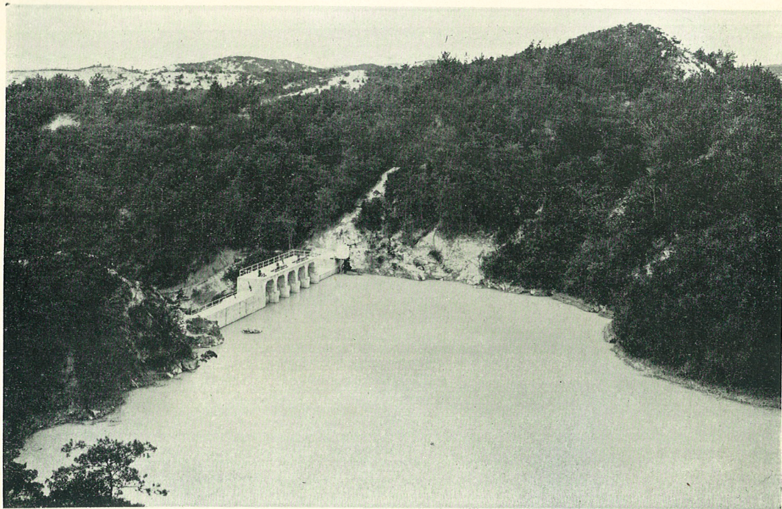
堰堤に依り流水を貯溜の状況 (第八頁記事参照)
