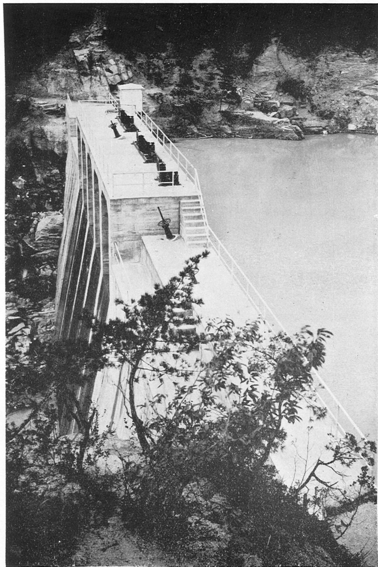
縮切堰堤の測面
