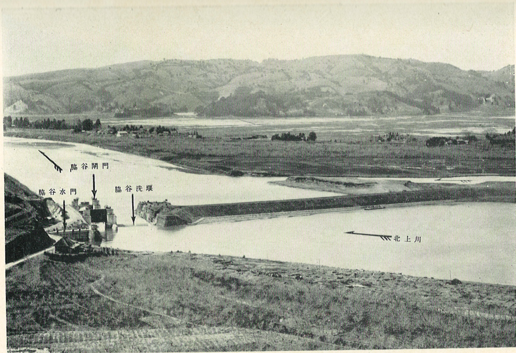
(1) 北上川締切箇所全景
