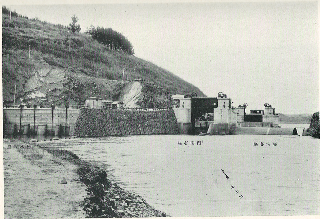
(2) 脇谷洗堰、脇谷閘門及脇谷水門
