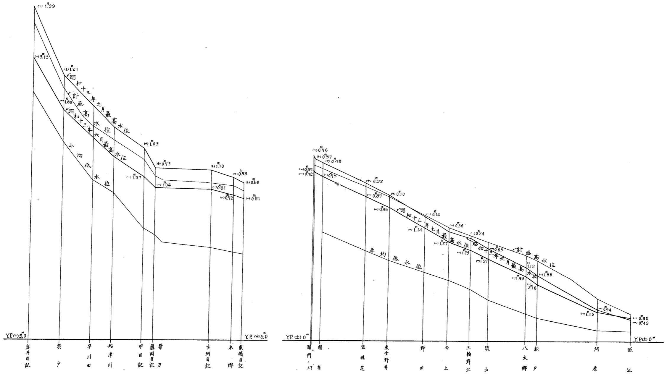
第九圖 利根川、渡良瀬川、江戸川最高水位縦断面圖
