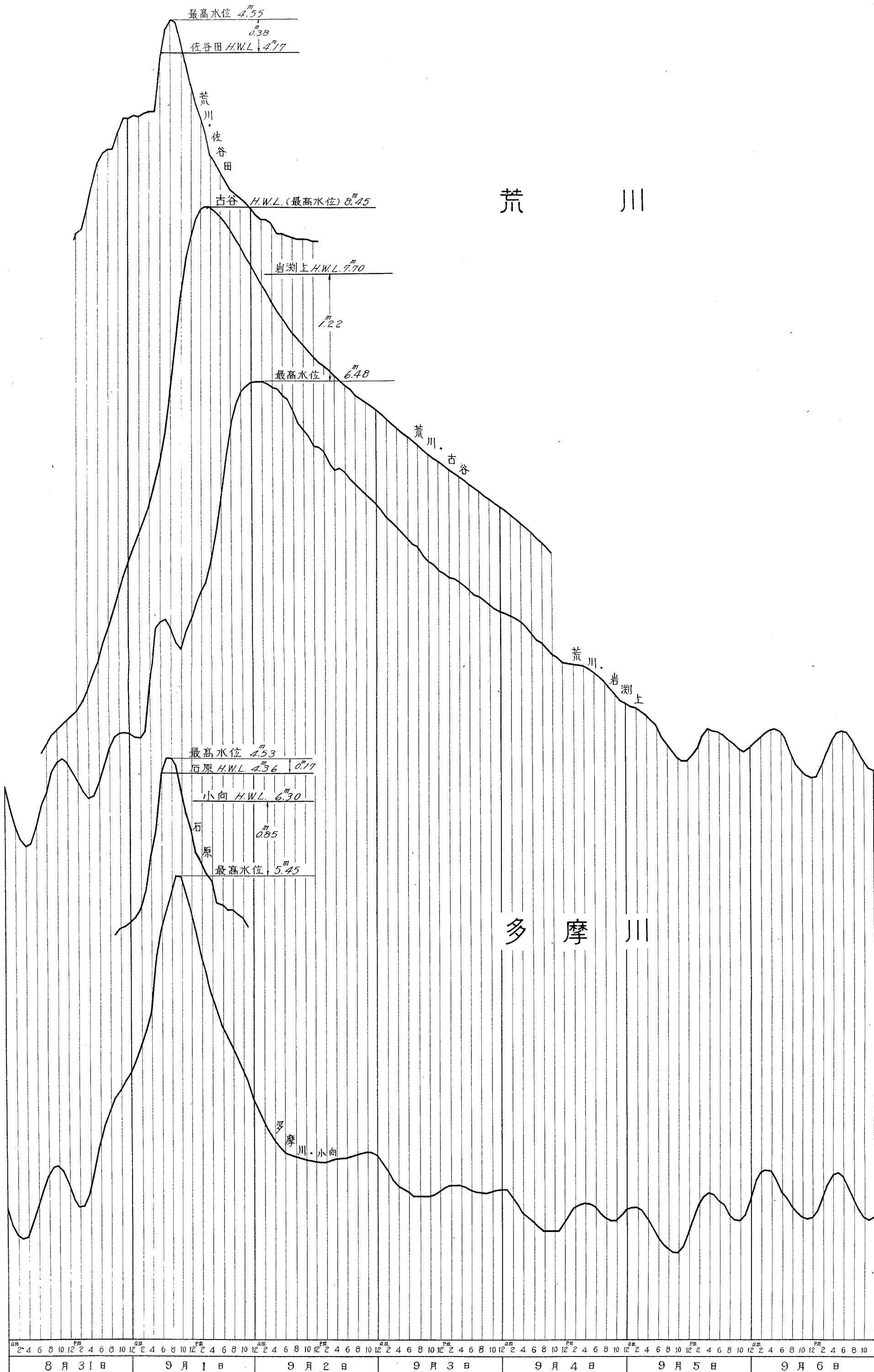
第八圖 昭和十三年八月下旬洪水 荒川多摩川水位曲線圖
