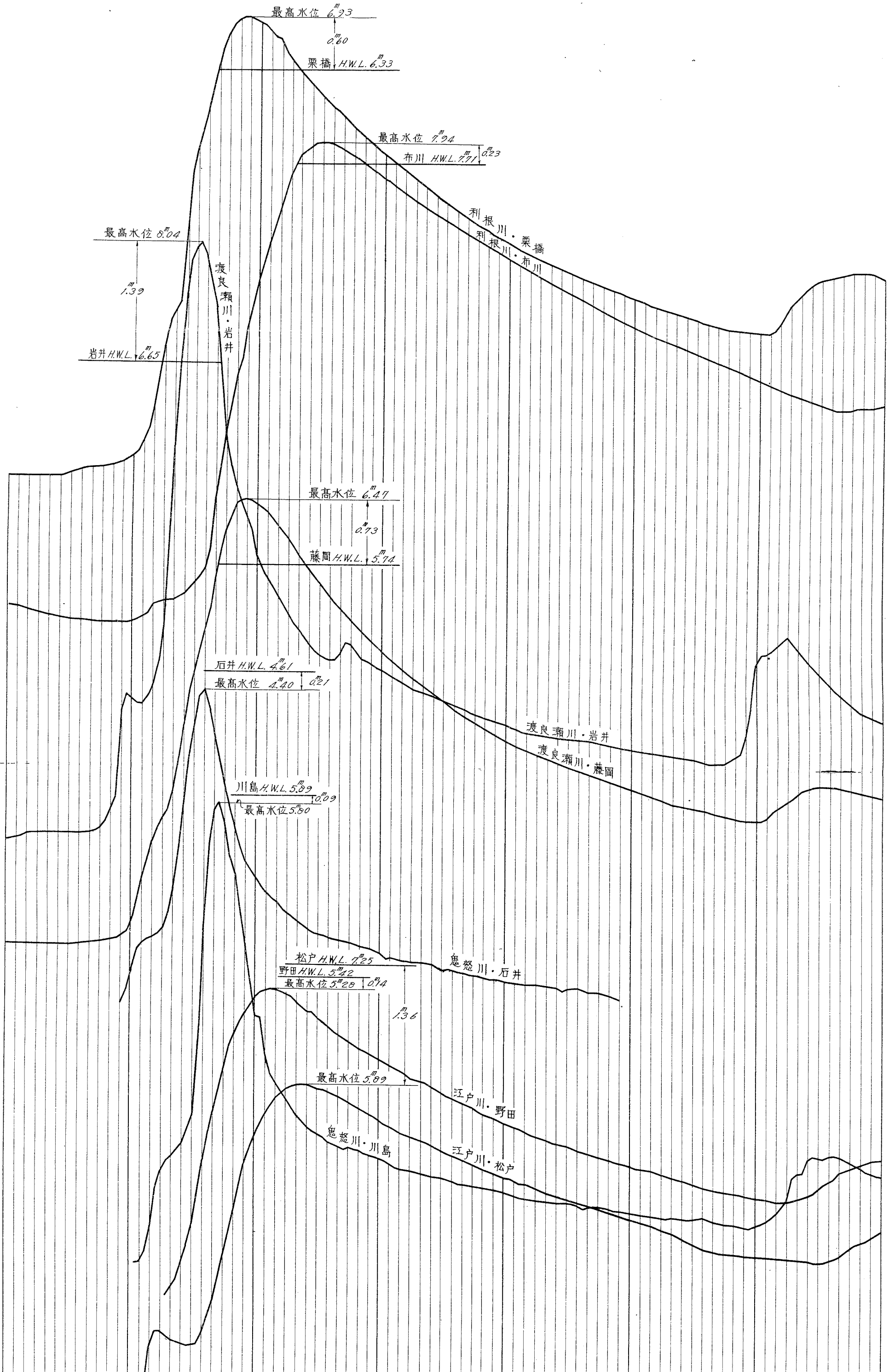
昭和十三年八月下旬 九月上旬洪水 利根川、渡良瀬川、江戸川、鬼怒川水位曲線圖
