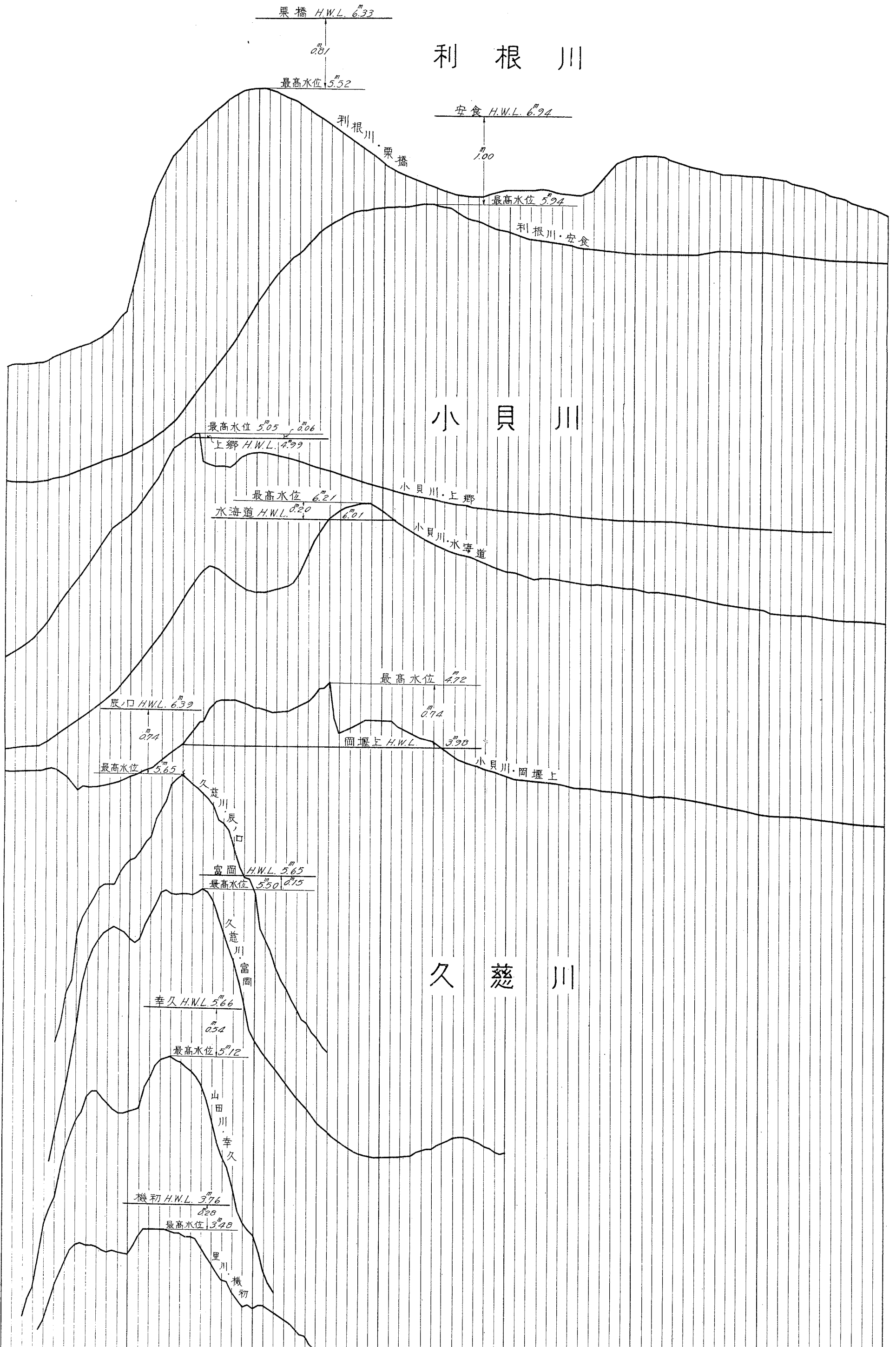
第五圖 昭和十三年六月下旬・七月上旬洪水 利根川、小貝川、久慈川水位曲線圖
