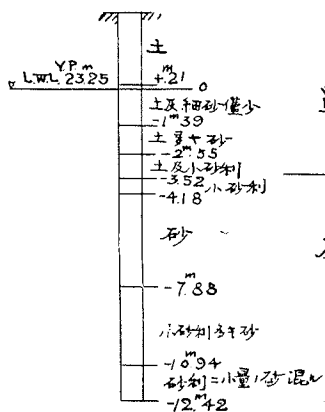
地質圖
