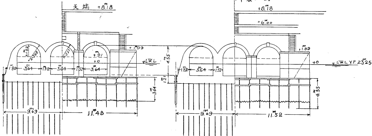
川裏正面
