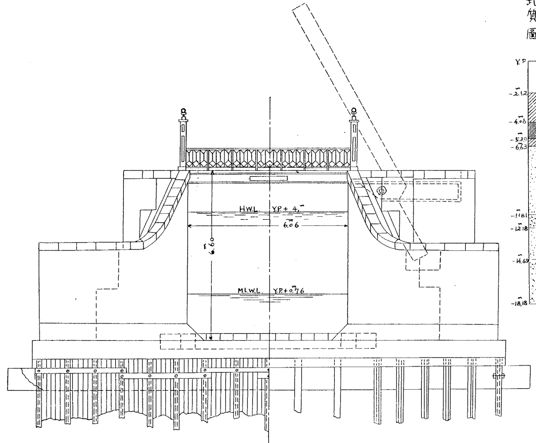
正面圖
