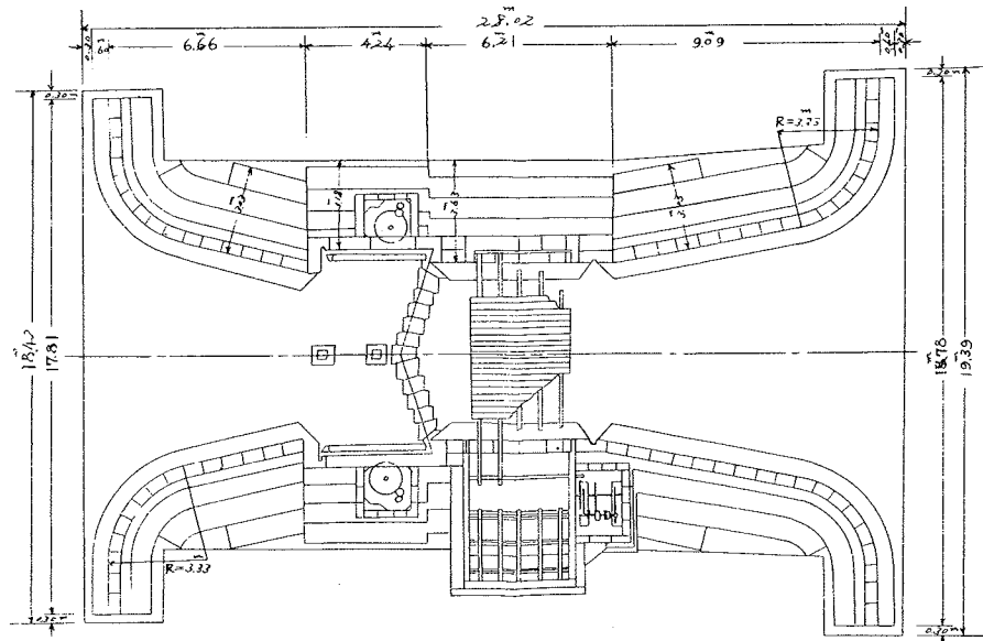
平面圖
