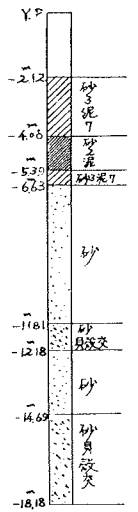
地質圖
