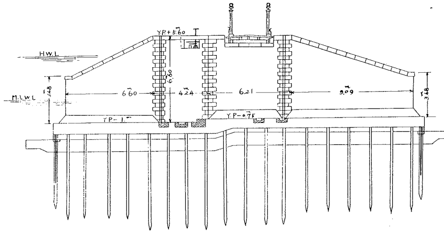
斷面圖
