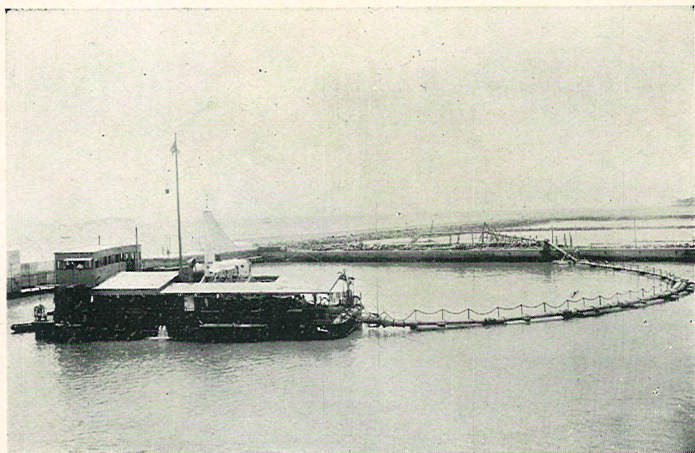
（用使號開開船潔浚式筒唧）業作立埋先地町崎州
