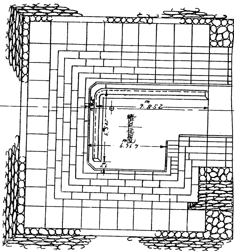
一般圖 縮尺二百分之一
