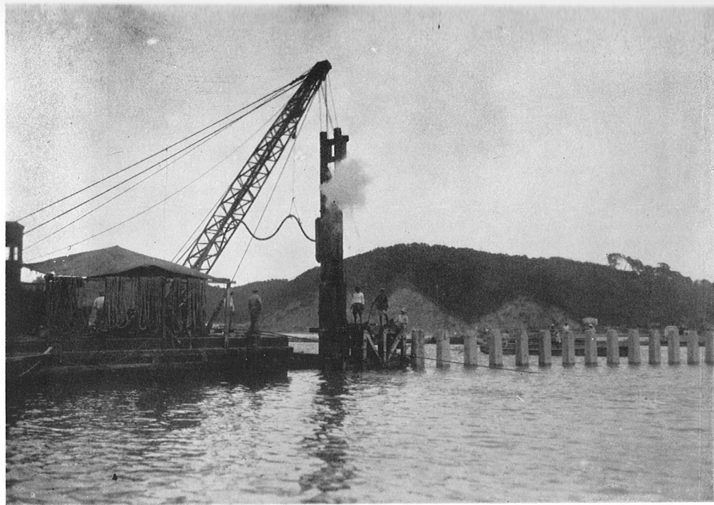
(5) 閉伊川左岸護岸鐵筋コンクリート杭打込作業
