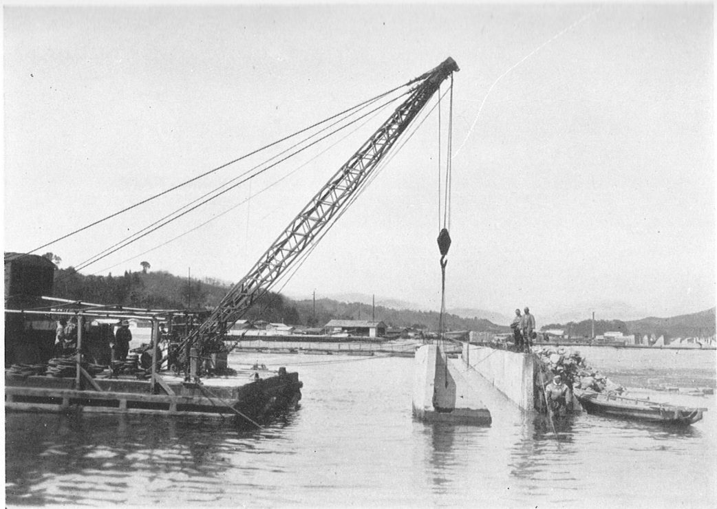
(4) 閉伊川左岸護岸L型塊据付作業
