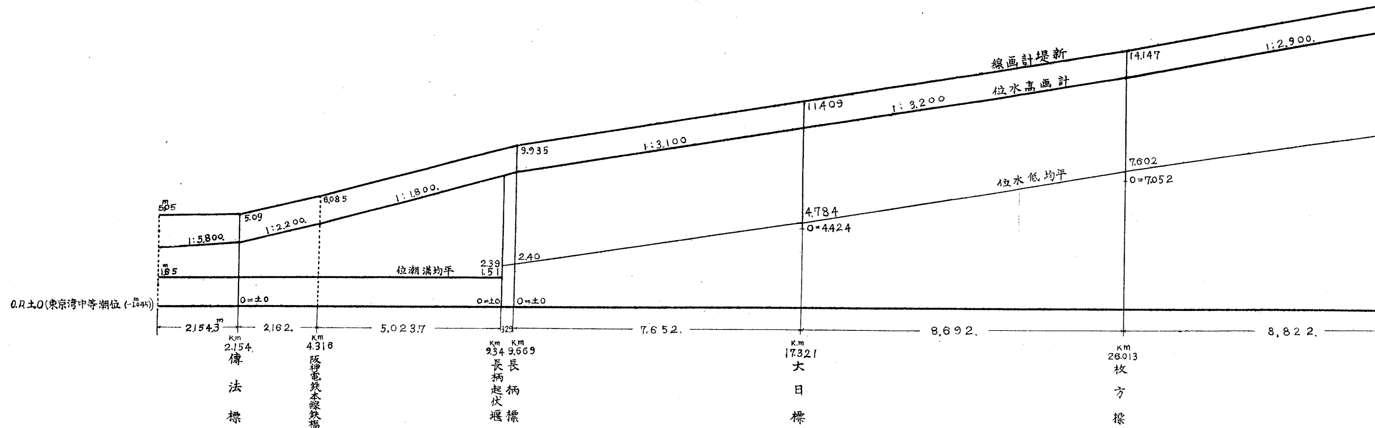
一之分百二尺縮 圖規定面斷防堤
