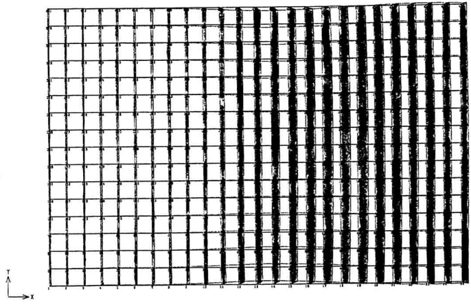
図-3 擬似3次元地盤モデルによる振動モード
