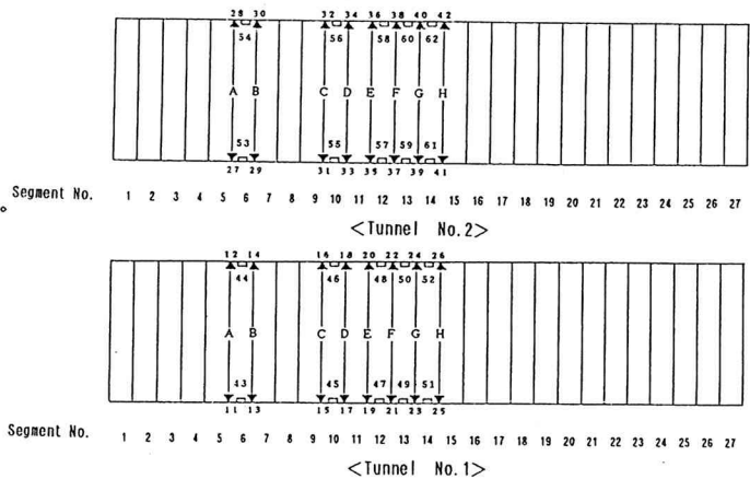
図-4 セグメント番号と測定断面
