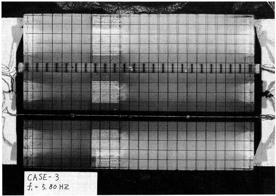
写真-1 CASE-3における模型共振時のプレ写真
