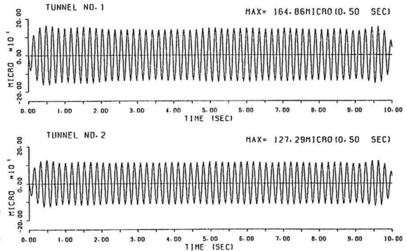
図-5 セグメント本体部ひずみ波形の比較
