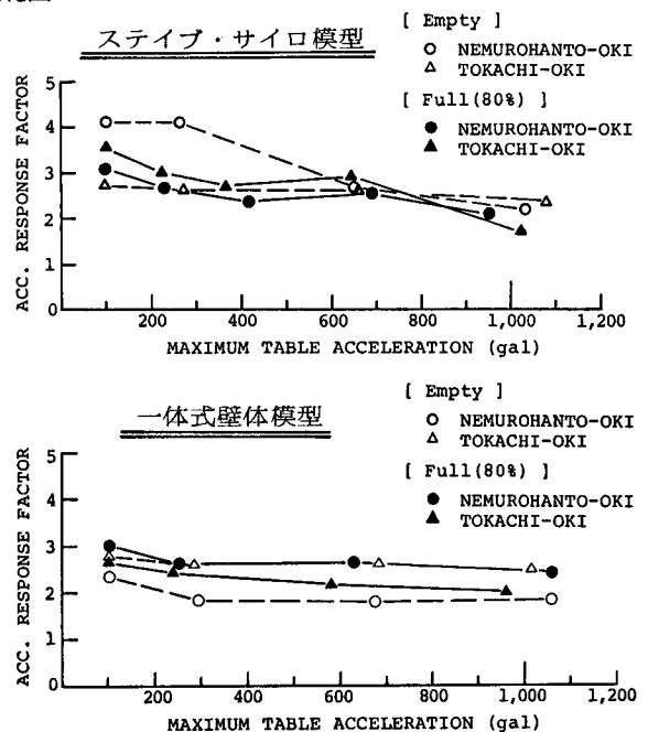
図4 入力加速度レベルの増大に伴う地震波応答倍率の推移の比較
