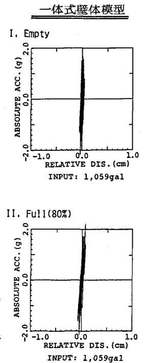
図8 地震波応答時復元力曲線の比較(根室半島沖地震波)
