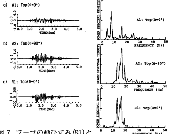
図7 フープの動ひずみ(R1)と加速度の応答性状(入力加速度約1,000galレベル)
