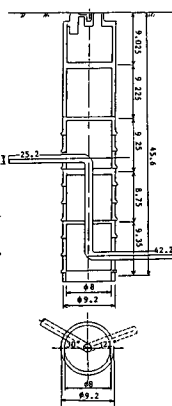
図1. 埋設構造物
