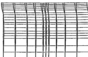
(b) 4次振動モード (固有振動数: 2.993 Hz, 寄与率: 21.20%)
