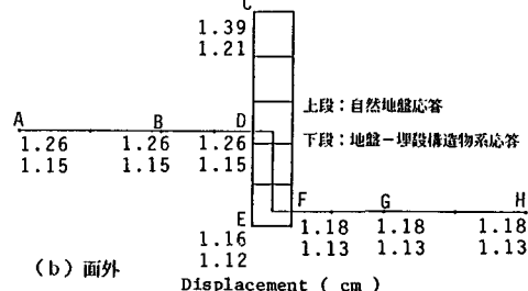
図5. 最大変位応答
