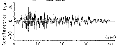
図2. 入力地震加速度波形 (伊豆東方沖地震・最大30gal)
