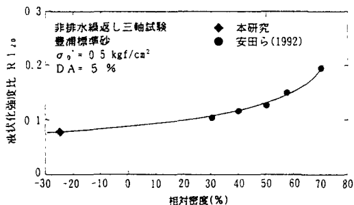
図6 液状化強度比と相対密度の関係
