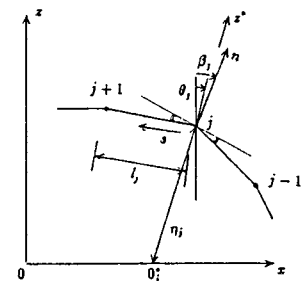
図-3 局所座標系
