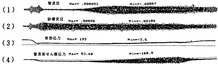
図2 管(軸方向)変位,砂槽変位,有効応力,管表面せん断応力の時刻歴(管理設深:-12cm)
