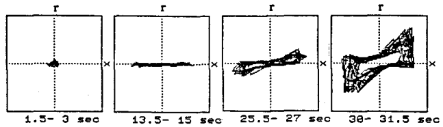
図3 管体復元力-相対変位曲線の例(管理設深:-12cm)
