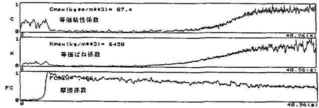
図4 管体復元力の等価粘性係数(c),等価ばね係数(k),摩擦係数(fc)の時刻歴(管理設深:-12cm)
