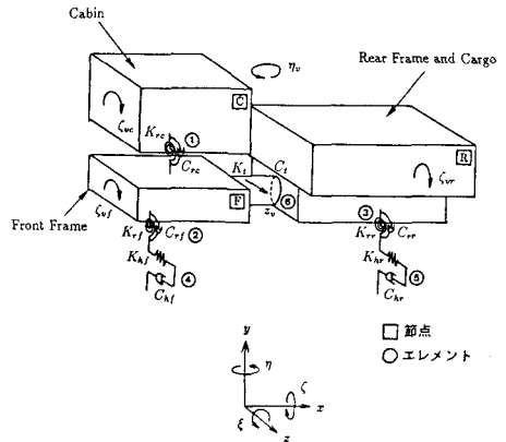
図-2 車両モデル
