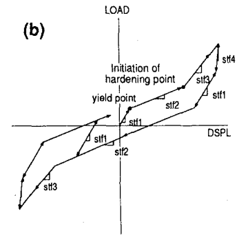
図-1 ハードニング履歴モデル
