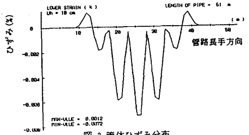
図-2 管体ひずみ分布
