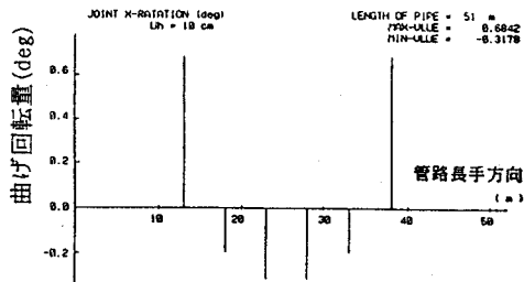
図-4 継手の曲げ回転
