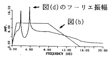
図-2 フーリエ振幅スペクトルの比較
