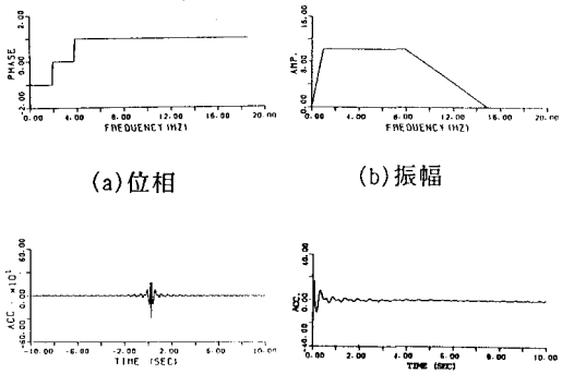
(a)位相 (b)振幅 (c)合成波形 (d) t < 0 の部分を0とした波形
