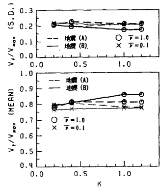
図3 盛土の耐震強化が危険列車の突入速度に与える影響
