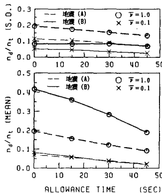
図4 減速余裕時間が列車危険度を与える影響
