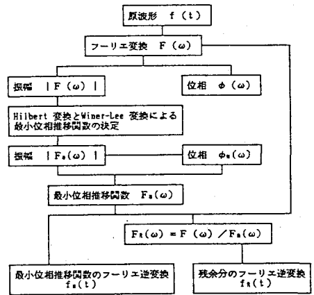
図-1 アルゴリズムのフローチャート
