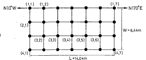
図3 1980年伊豆半島東方沖地震の断層を小分割したモデル
