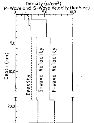
図2 伊豆半島付近の地下構造
