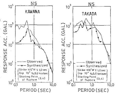
図6 観測波形と理論波形による加速度応答スペクトルの比較
