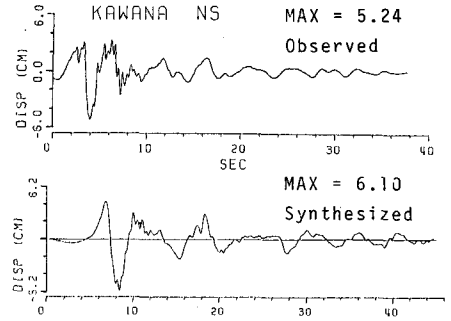
図4 川奈における観測および理論変位波形
