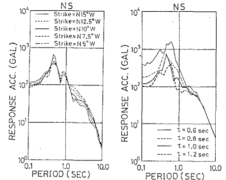
図7 走向と rise time の変化が加速度応答スペクトル(川奈 NS)に及ぼす影響
