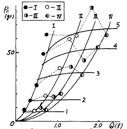
図-3 動水圧と貯水量の関係
