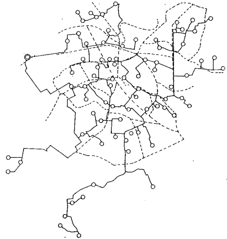
2. T地区中圧管路網図
